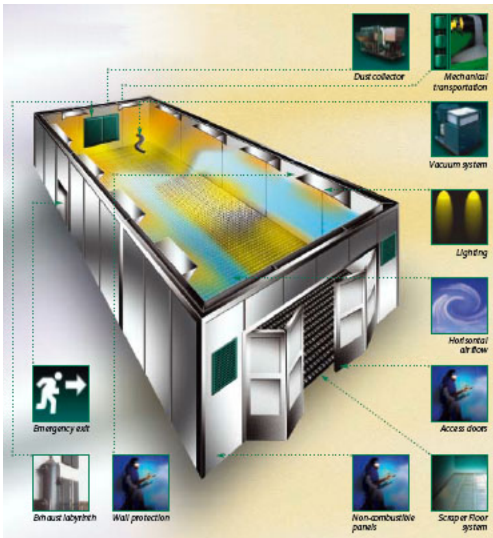
Størrelsen på kabinen dimensjoneres etter kundens ønske. Bildet viser en kabin med følgende mål L x B x H = 13,2 x 6,6 x 4 m.
